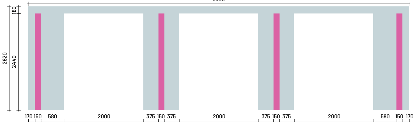
Binnen aanzicht
