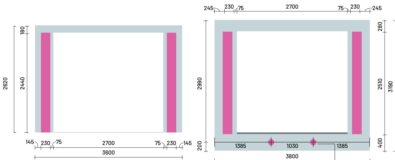
Binnen aanzicht
