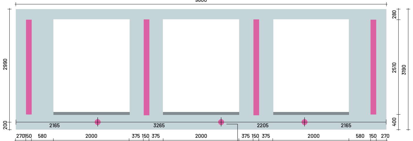
Buiten aanzicht
