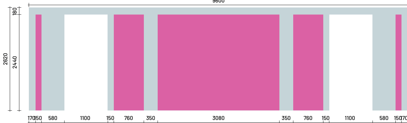
Buiten aanzicht
