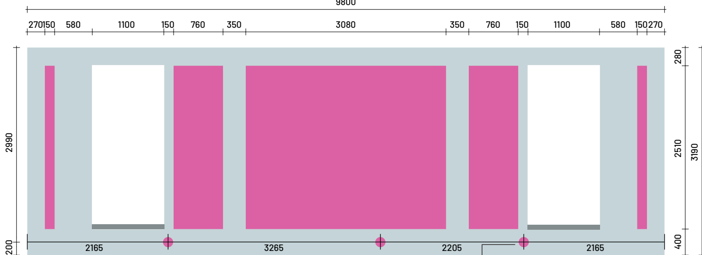
Buiten aanzicht
